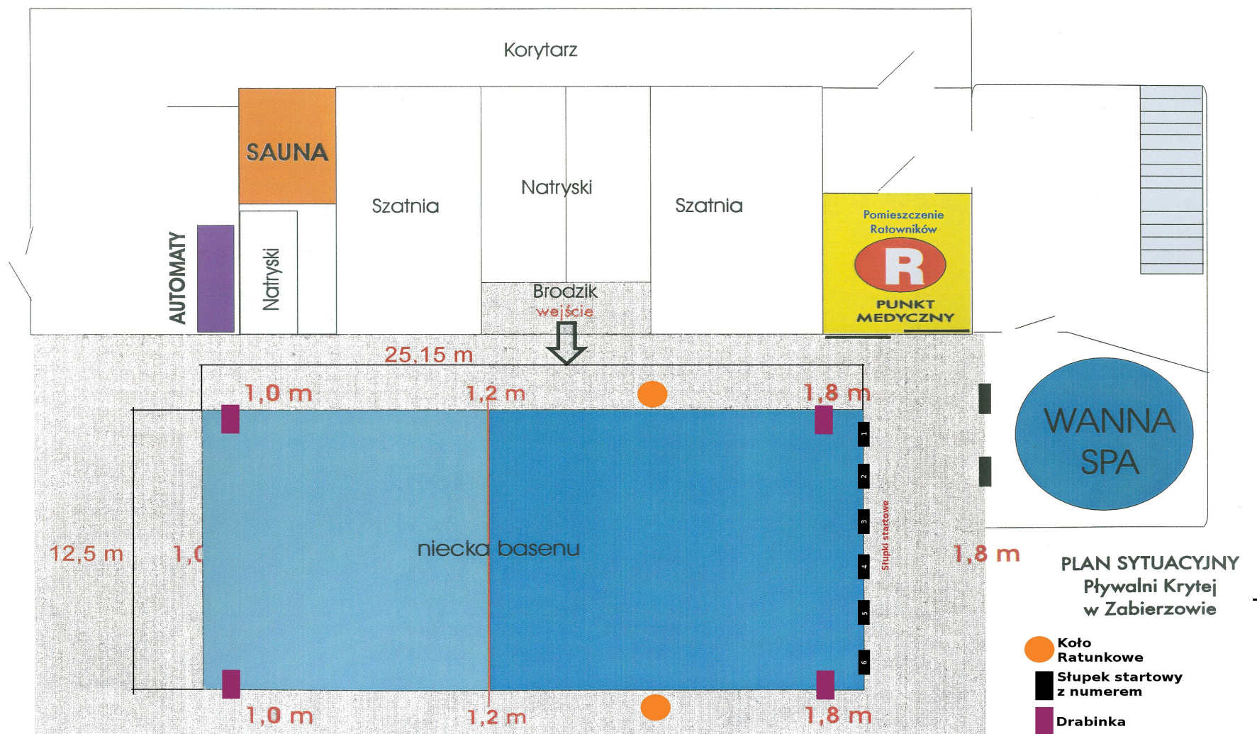
Rysunek 1. Schemat pływalni wraz z rozkładem głębokości
